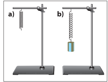
2.6. Deformarea resortului
